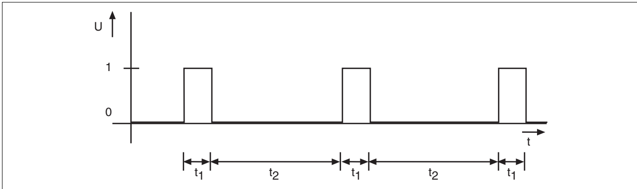
Zeitdiagramm
