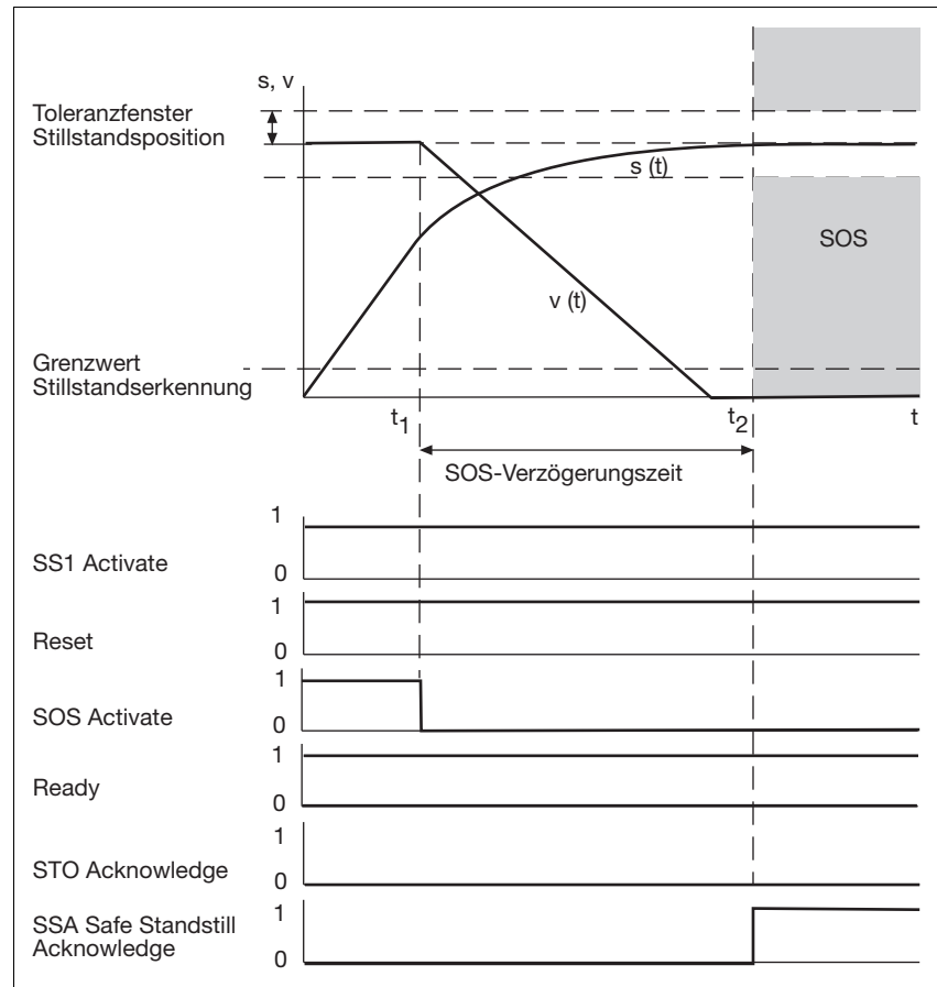
Fig. 4-6: Sicherheitsfunktion SOS
