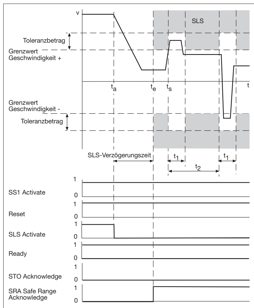
Fig. 4-8: Sicherheitsfunktion SLS mit aktivierten Toleranzbereich
