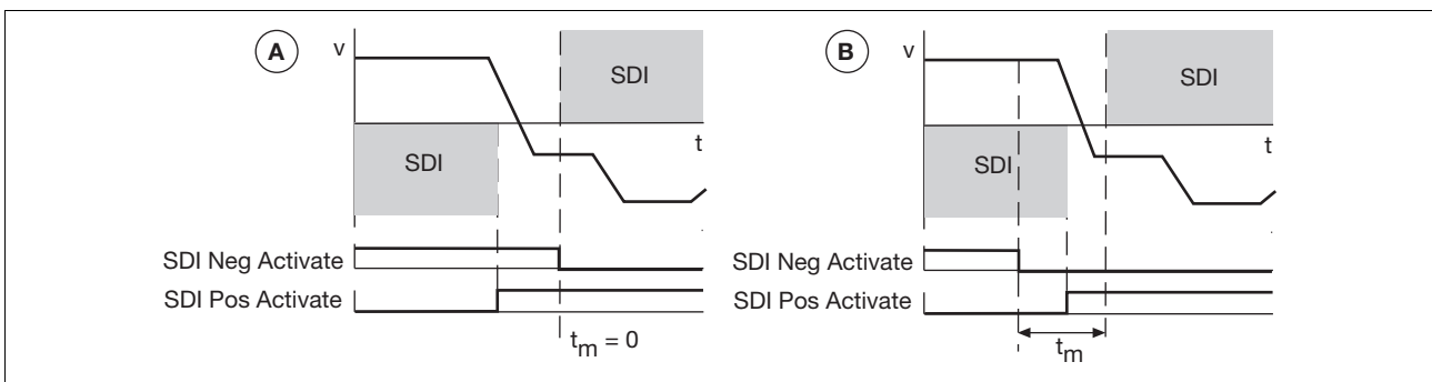
Fig. 4-12: Änderung der Drehrichtung
