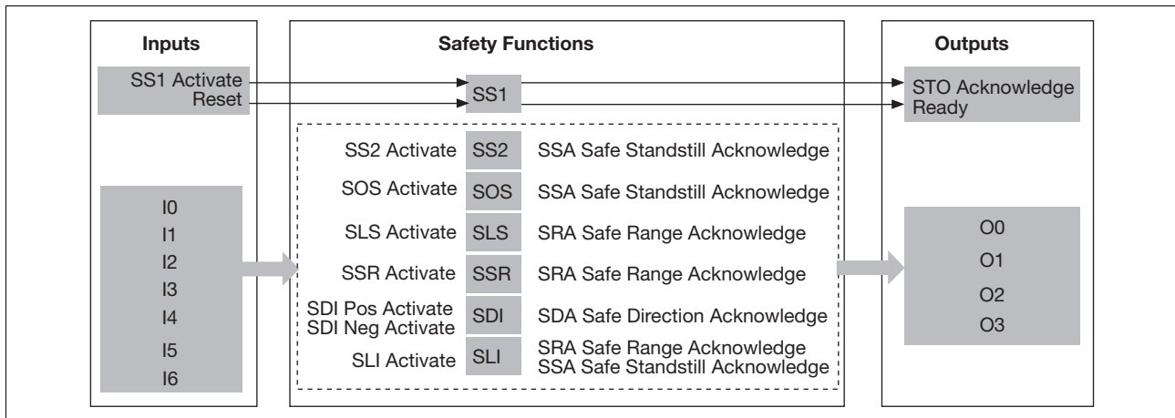
Fig. 4-2: Ein- und Ausgänge
