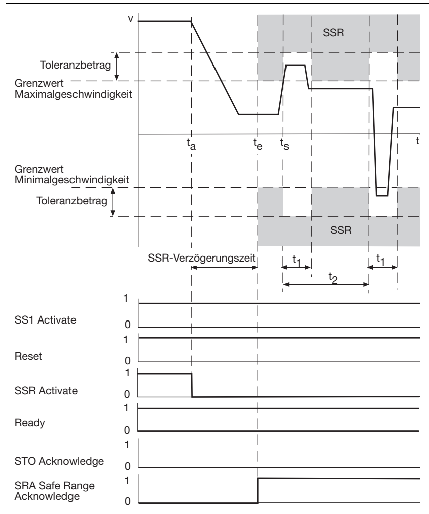
Fig. 4-10: Sicherheitsfunktion SSR mit aktivierten Toleranzbereich ▶ Toleranzbetrag in % der beiden Grenzwerte Maximal- und Minimalgeschwindigkeit ▶ t_a : Auslösung der Sicherheitsfunktion SSR ▶ t_e : nach Ablauf der SSR-Verzögerungszeit Überwachung der Geschwindigkeit ▶ t_s : Geschwindigkeit v überschreitet Grenzwert und aktiviert den Toleranzbereich (Toleranzbetrag, Toleranzzeit, Toleranzperiode) ▶ t_1 : Toleranzzeit ▶ t_2 : Toleranzperiode ▶ SS1 Activate: Eingang für Sicherheitsfunktion SS1 ▶ Reset: Eingang für Reset ▶ SSR Activate: Eingang für Sicherheitsfunktion SSR
