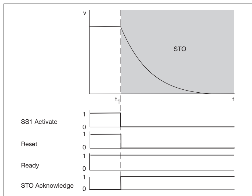
Fig. 4-3: Sicherheitsfunktion STO
