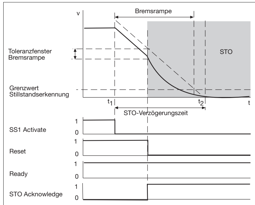
Fig. 4-4: Sicherheitsfunktion SS1
