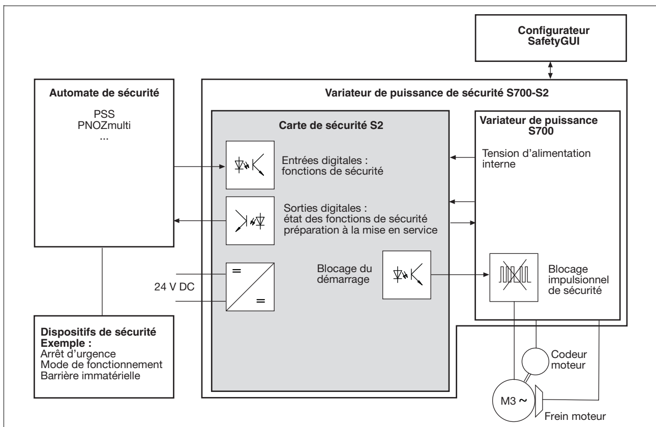
Fig. 4-1: Système d'entraînement de sécurité
