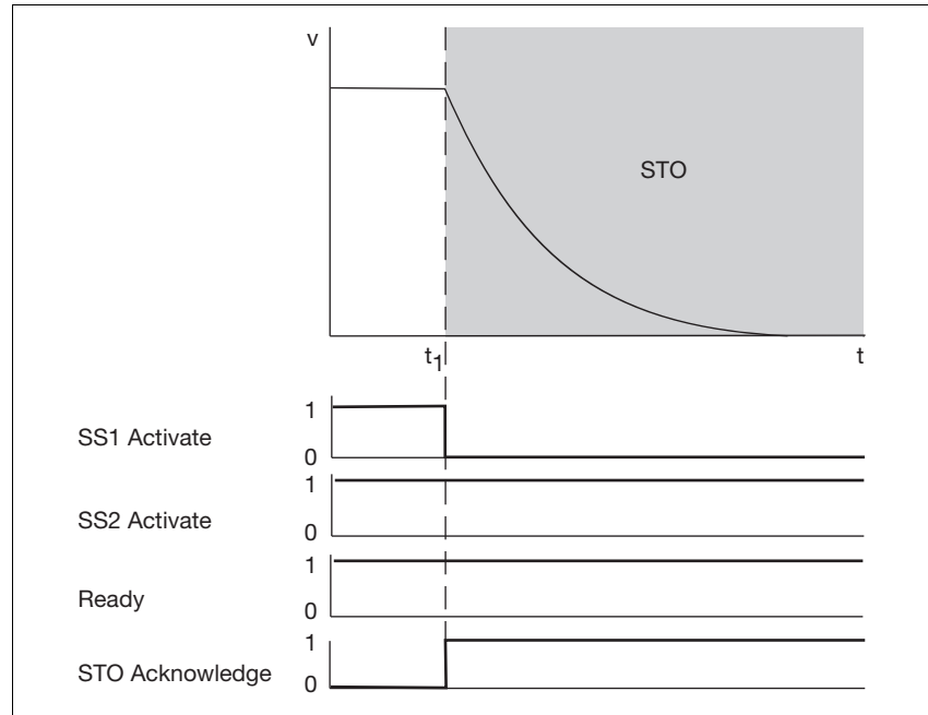
Fig. 4-2: Fonction de sécurité STO
