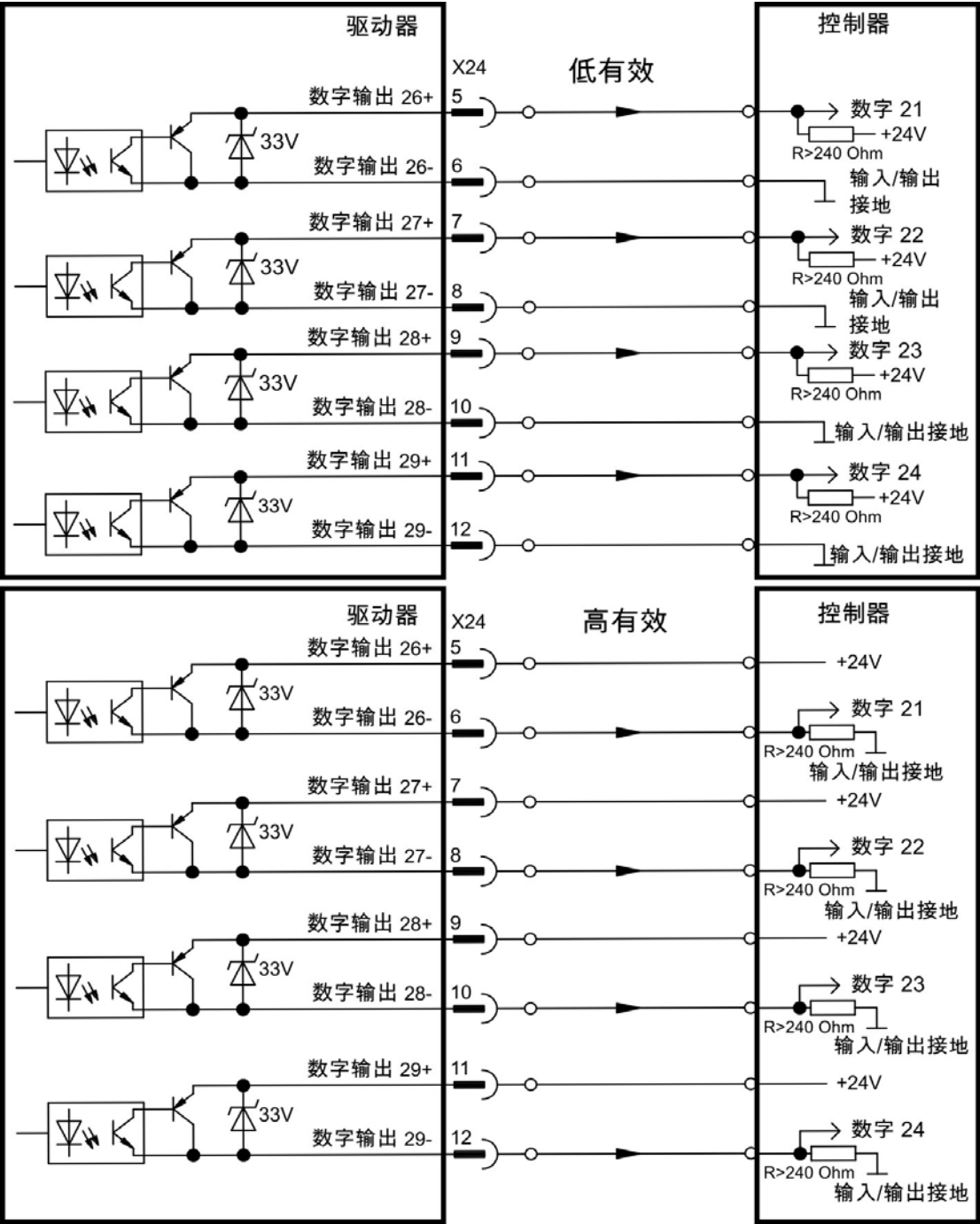
接线图 X24
