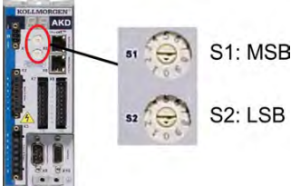
将 S1 设置为 8，将 S2 设置为 9
