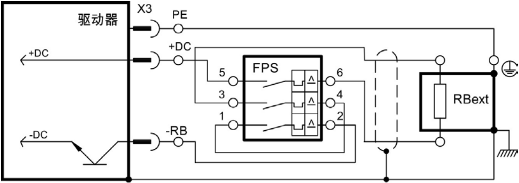
FPS:Frizlen 直流电源开关
