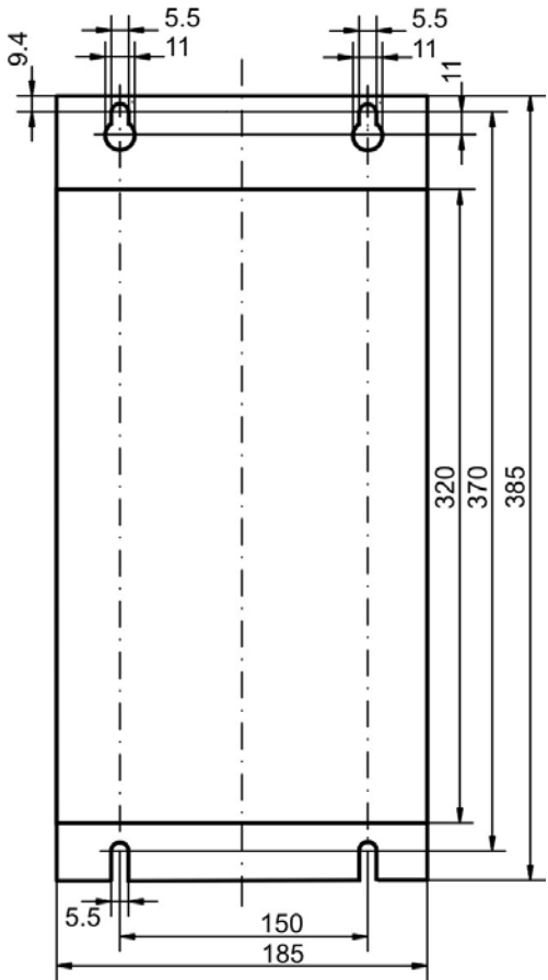
AKD 加长宽度 480V, 48A
