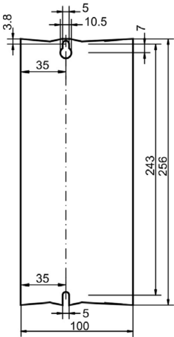
AKD 加长宽度 480V, 3A 至 12A
