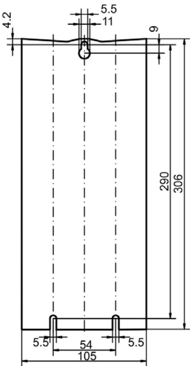
AKD 加长宽度 480V, 24A
