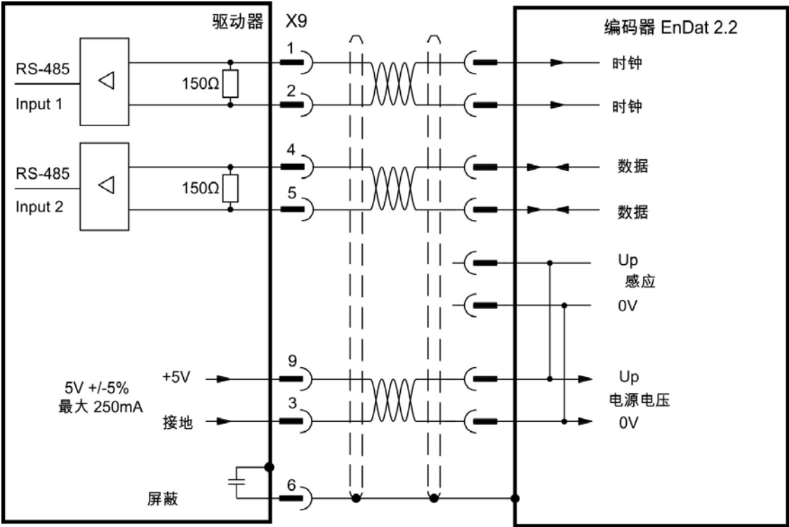
连接图
