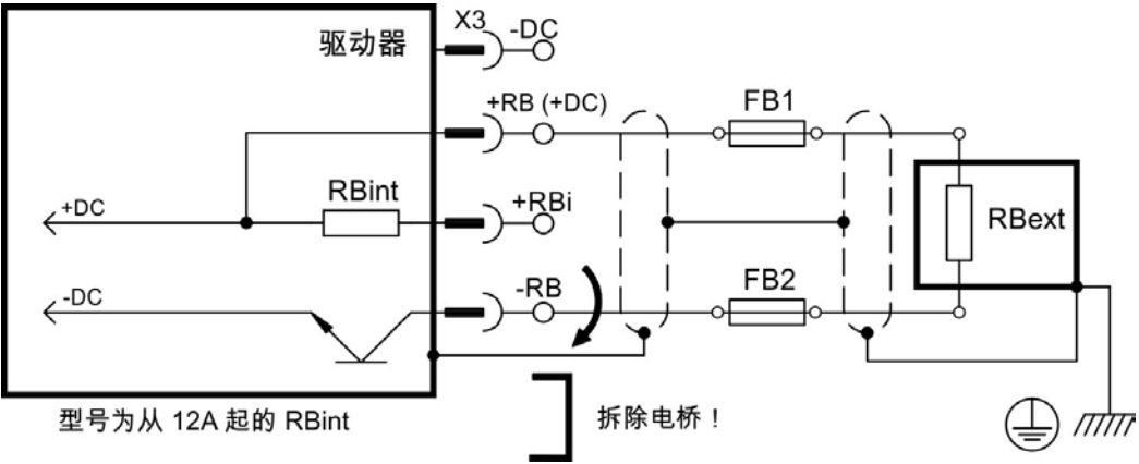
FB1 / FB2 保险功能
