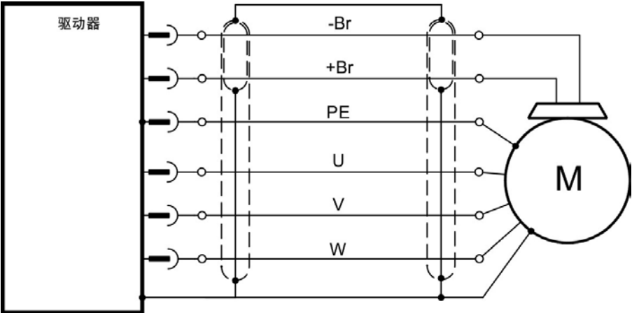
电缆长度 >25 m
