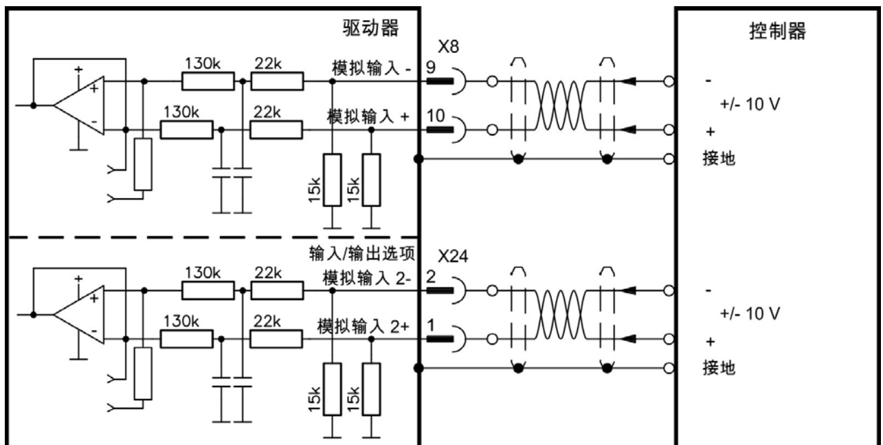
模拟输入接线图
