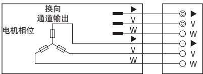
电机连接
