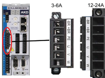
图 4. 连接器 X2, AKD-xxxx06
