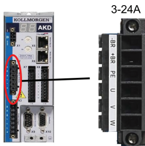
图 5. 连接器 X2, AKD-xxxx07
