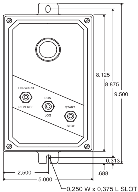
BVFD163 & BVFD163WD DIMENSIONS
