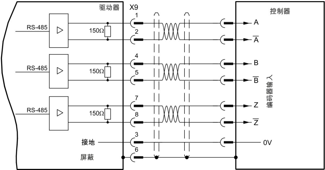
连接图
