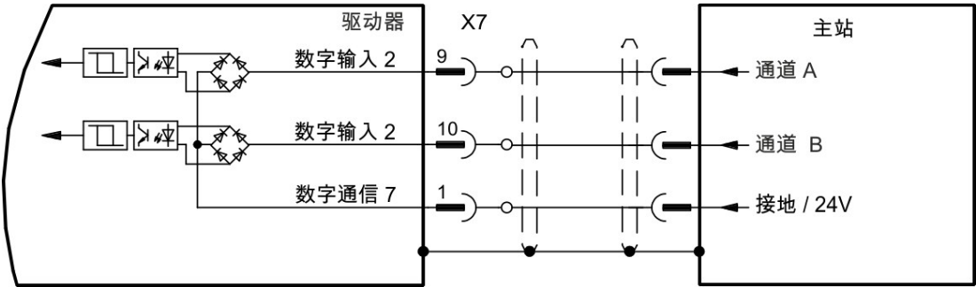
连接图
