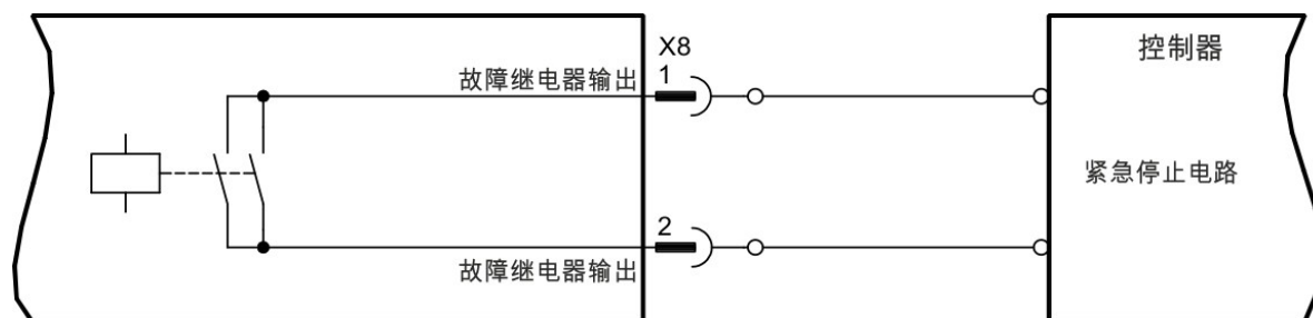
接线图
