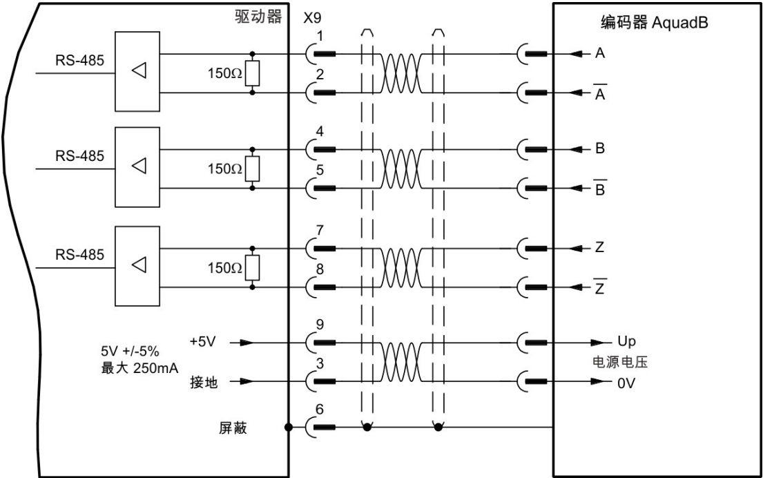
连接图
