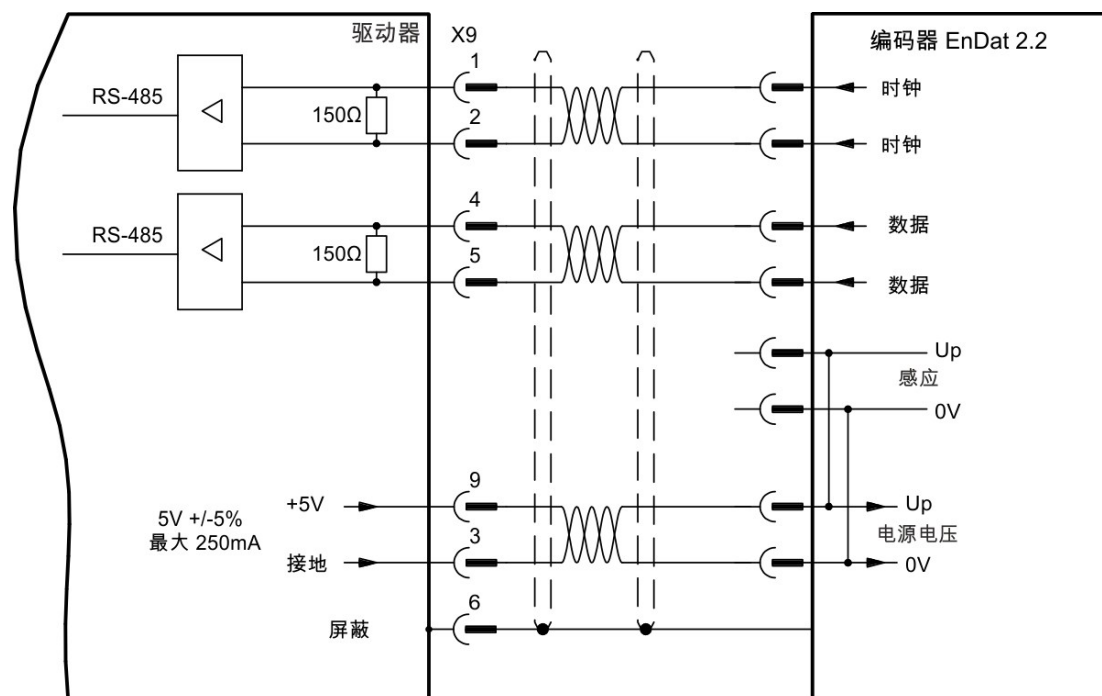
连接图
