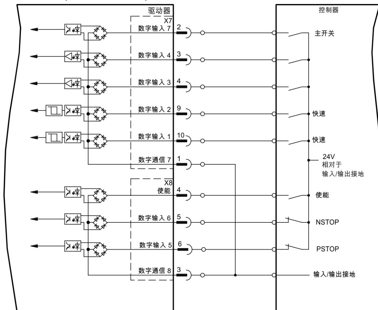
数字输入接线图(例如，共源类型连接)
