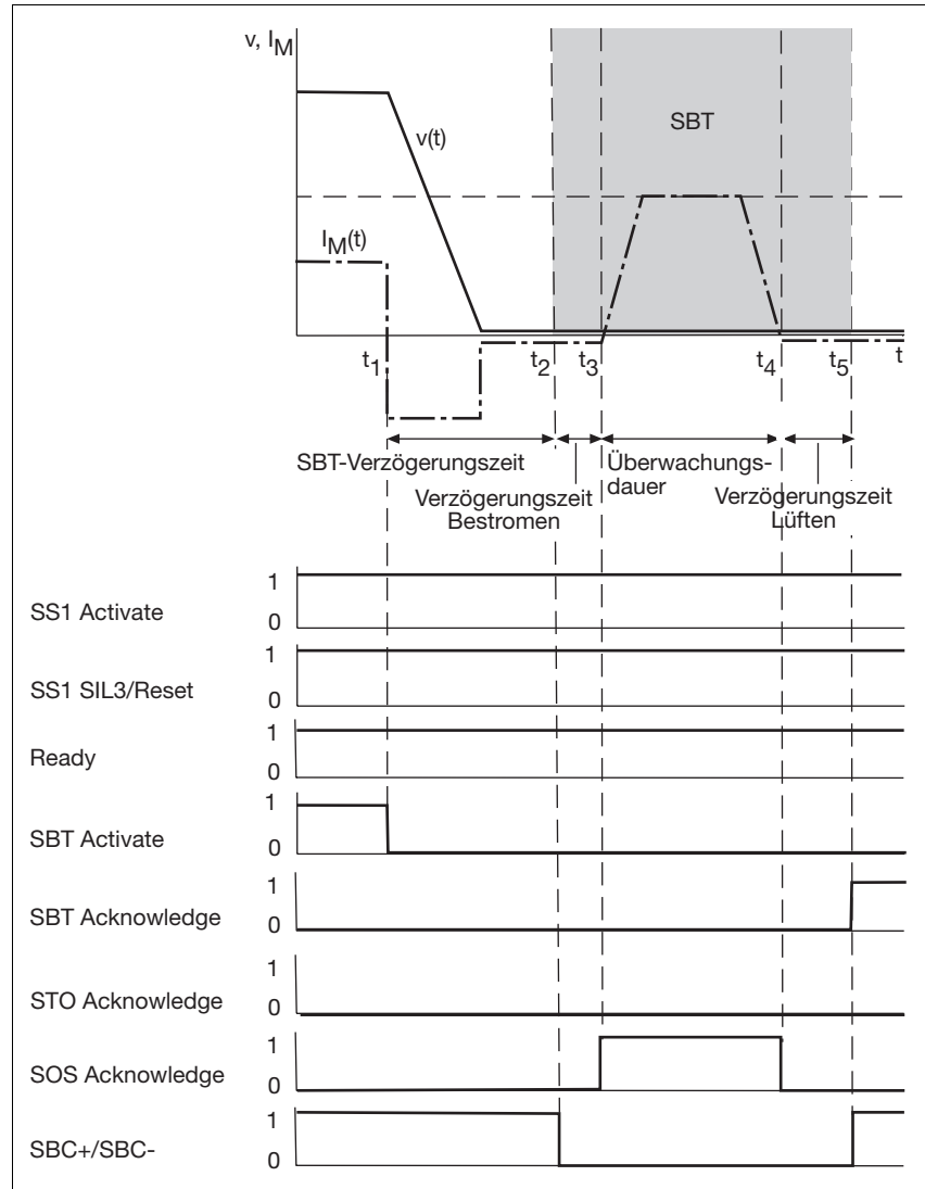
Fig. 4-14: Sicherheitsfunktion SBT
