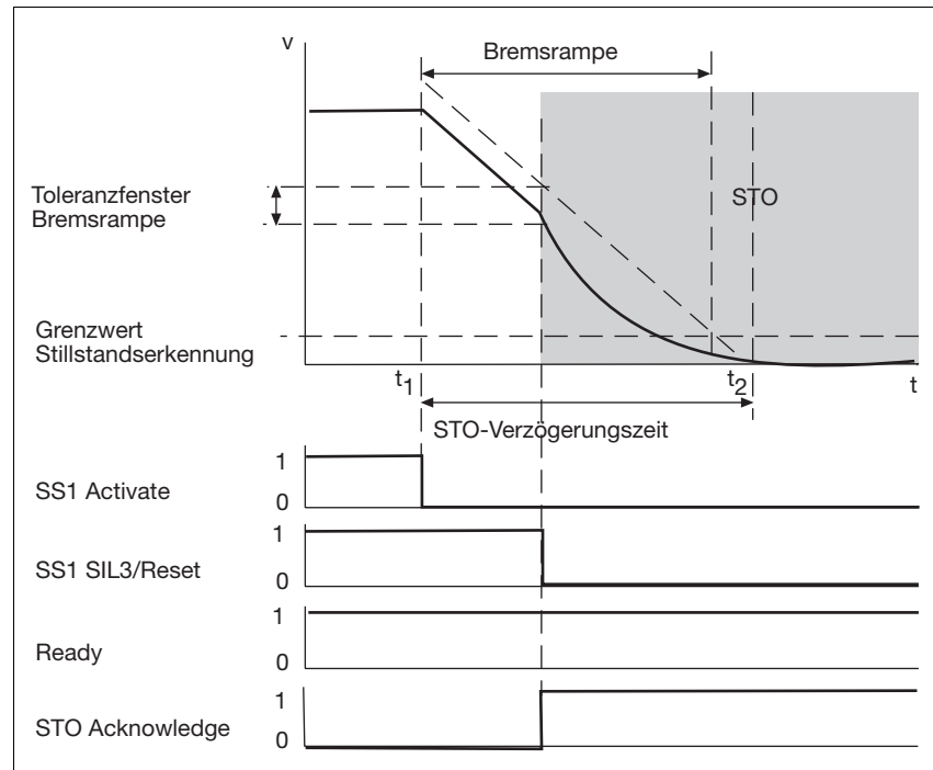
Fig. 4-3: Sicherheitsfunktion SS1
