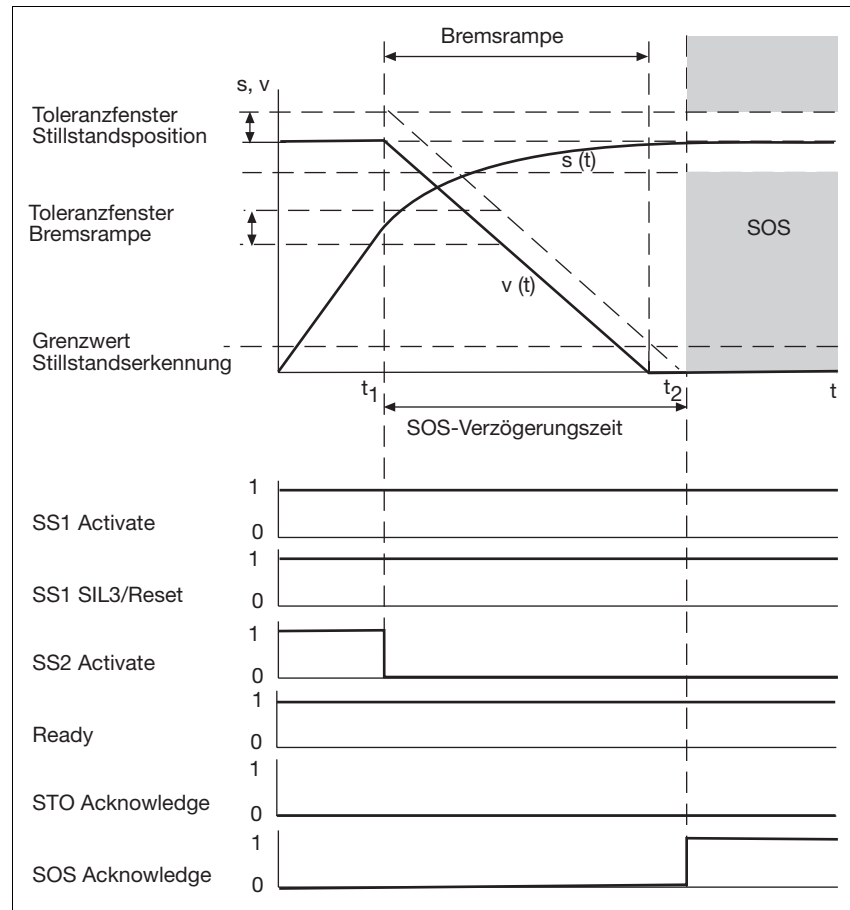
Fig. 4-4: Sicherheitsfunktion SS2
