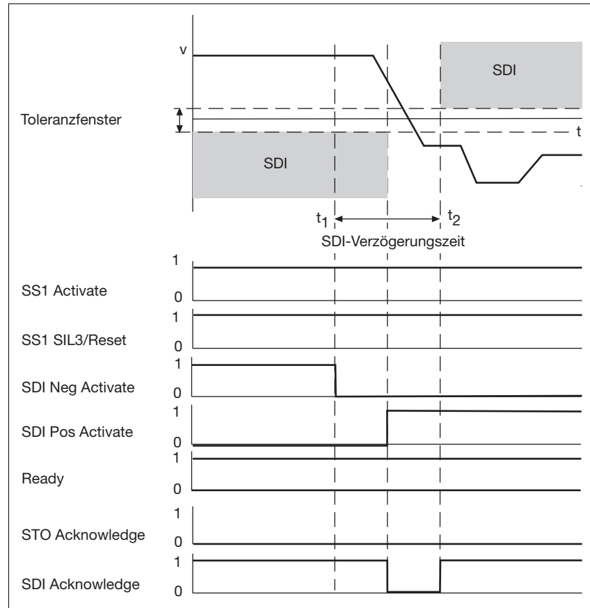
Fig. 4-12: Änderung der Drehrichtung mit SDI-Verzögerungszeit
