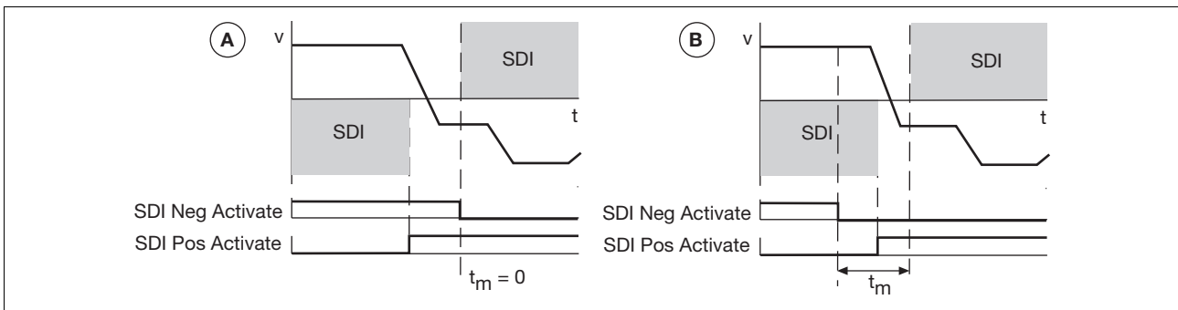
Fig. 4-11: Änderung der Drehrichtung
