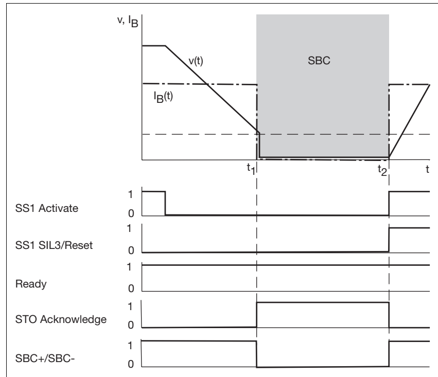
Fig. 4-13: Sicherheitsfunktion SBC
