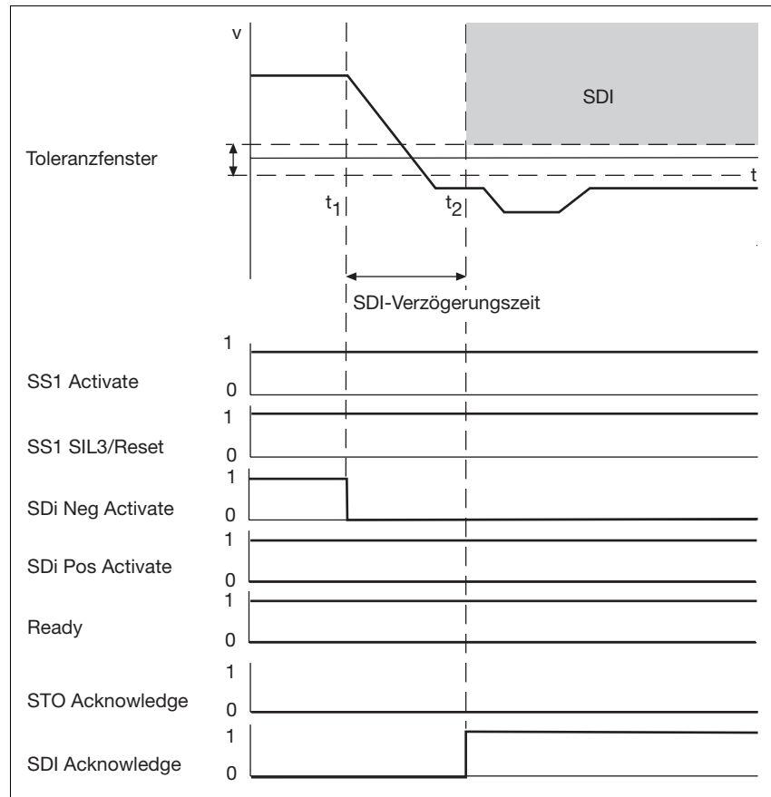
Fig. 4-10: Sicherheitsfunktion SDI
